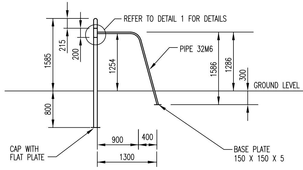
END ELEVATION
