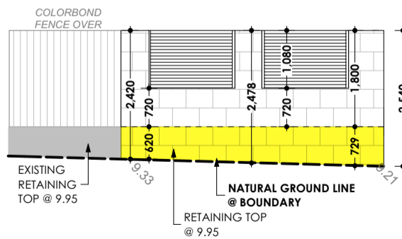
ELEVATION 3 1:100
