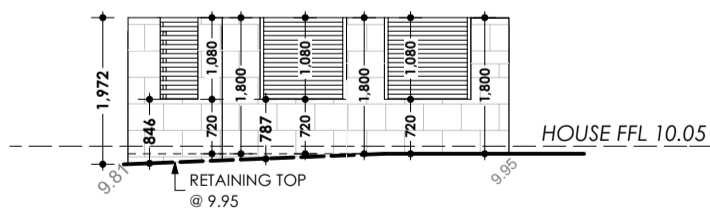
ELEVATION 2 1:100
