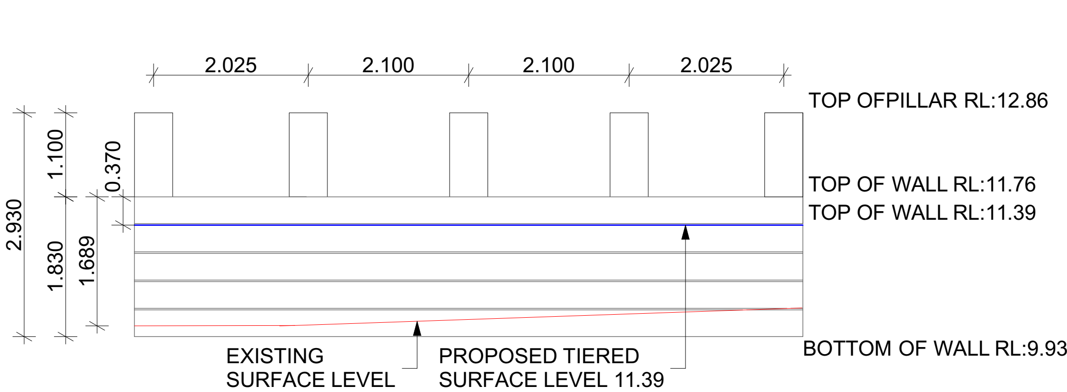
Elevation 1
