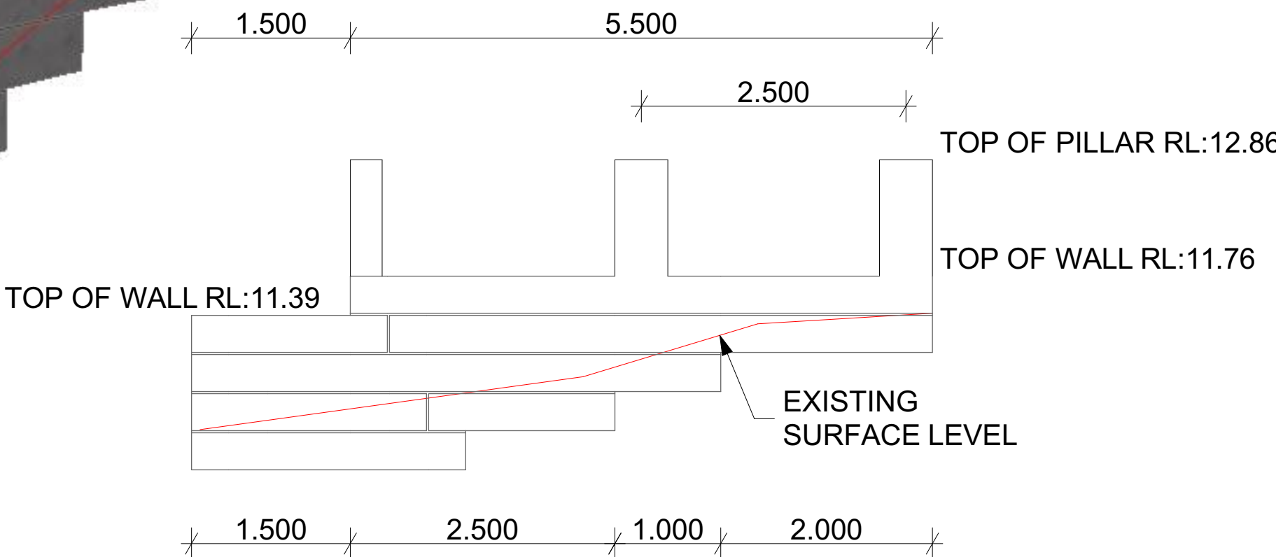
Elevation 2
