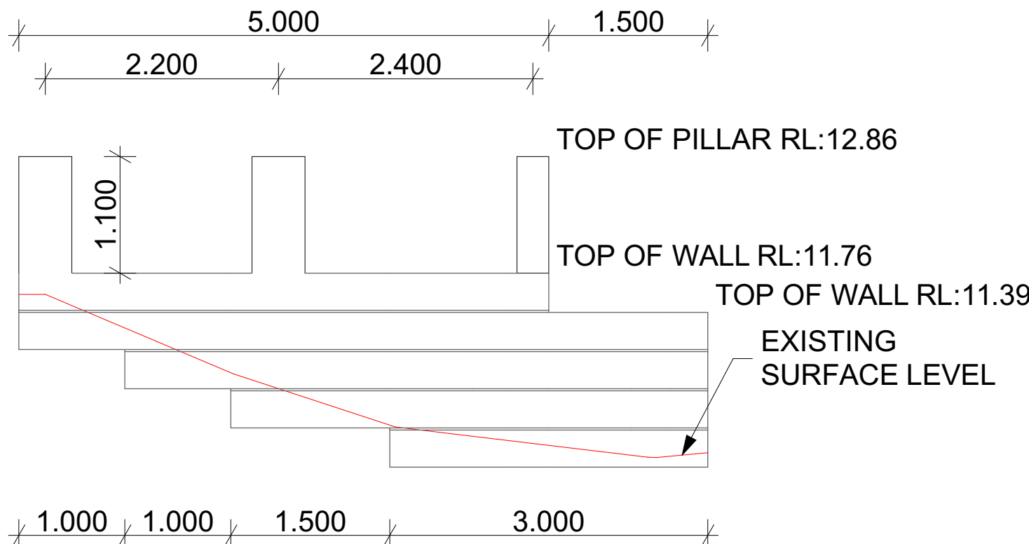
Elevation 3
