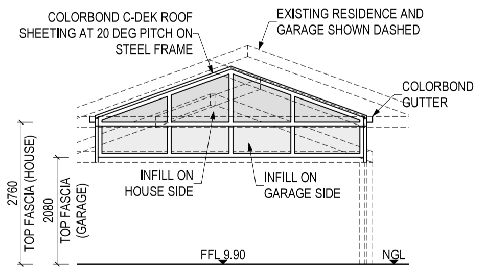
SECTION - PATIO Scale: 1:75
