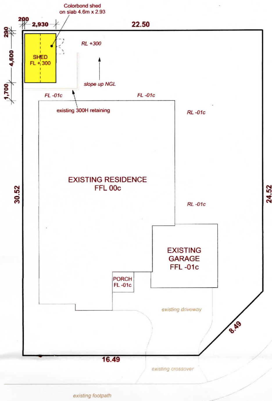
SITE PLAN 1:200
