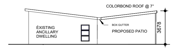
ELEVATION 3 1:100
