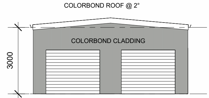
ELEVATION 1 1:100
