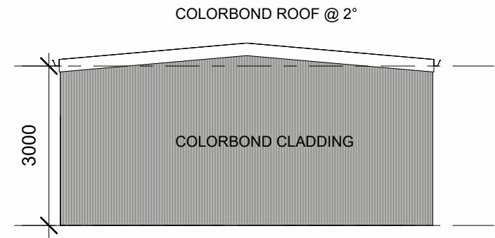
ELEVATION 3 1:100
